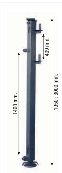
COLUMNA P / P COLUMN
