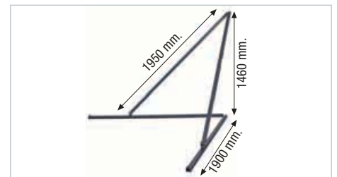
BÍPODE / BIPOD
