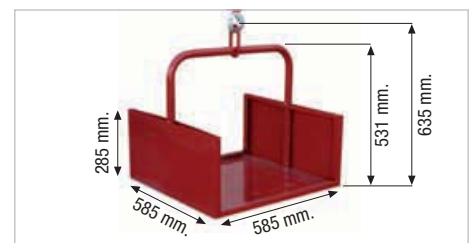
JAULA / METAL CAGE
