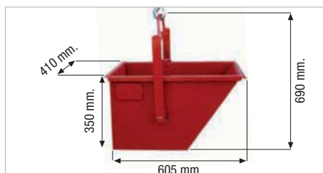
CUBILOTE / BUCKET
